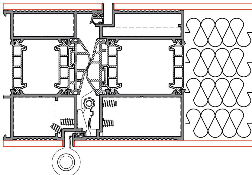
Схема на профила за премиум входни врати
