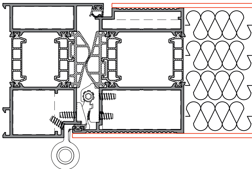
Схема на профила за входни врати
